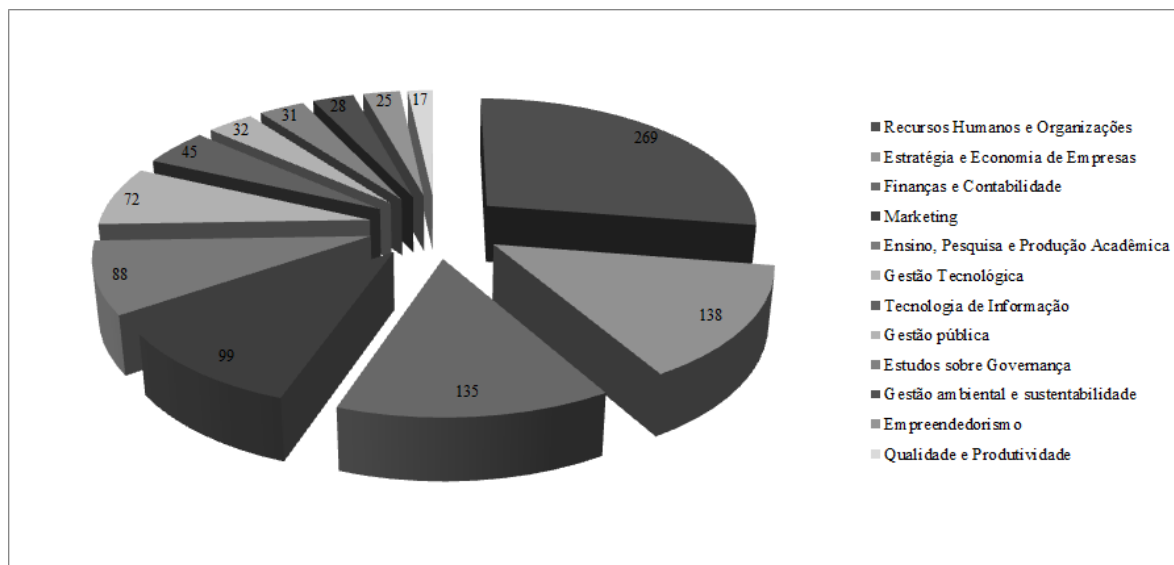
Gráfico 7 - Áreas temáticas
