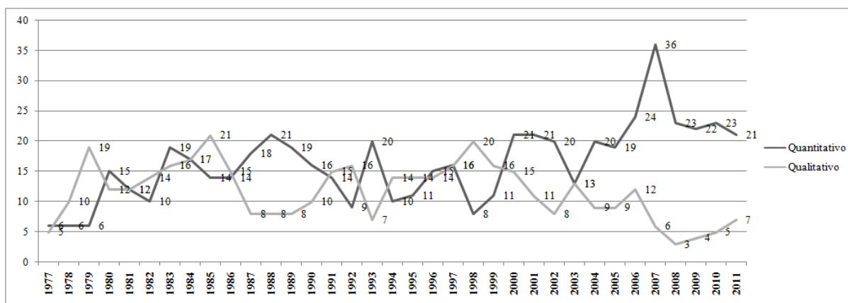
Gráfico 6 - Abordagens metodológicas
