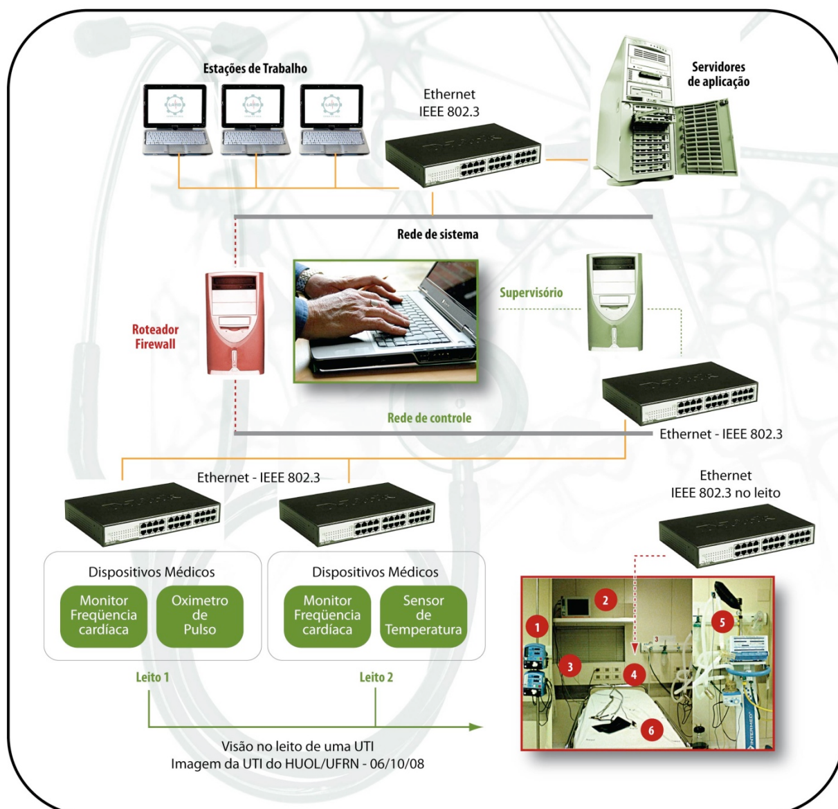
Figura 2 - Modelo Arquitetural de Rede Aplicada na Automação Hospitalar
