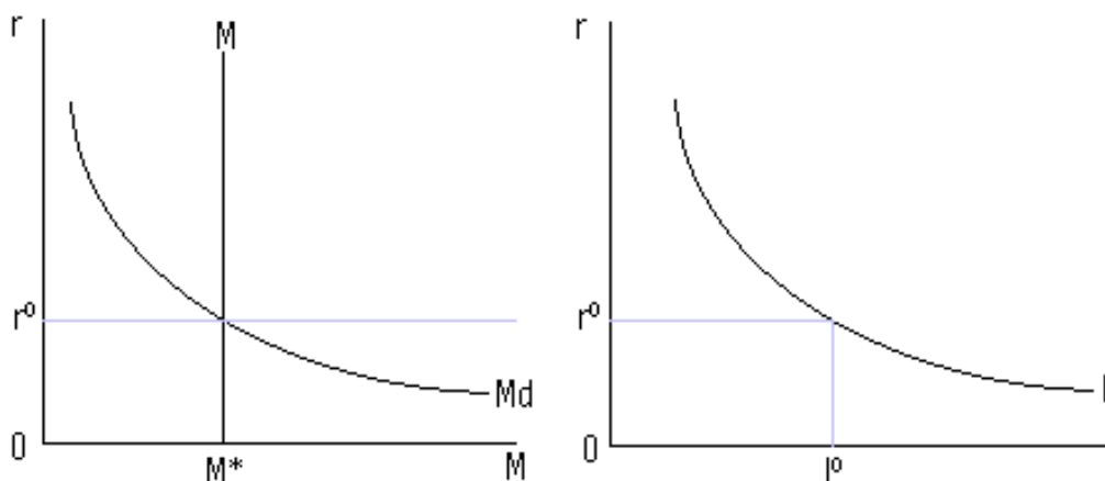
Gráfico 02: taxa de juros e eficiência marginal do capital.
