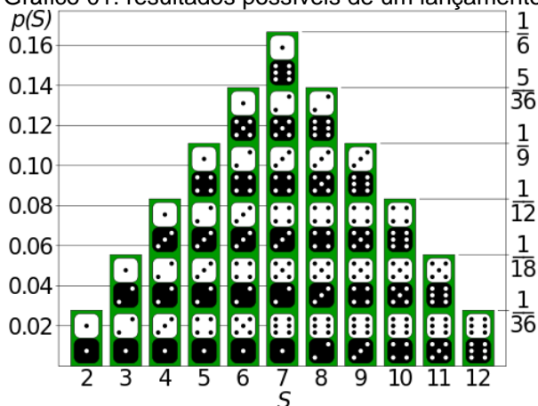
Gráfico 01: resultados possíveis de um lançamento de dois dados simultaneamente.
